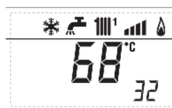
32. zobrazení relé R2 na solárním okruhu (INSOL)
