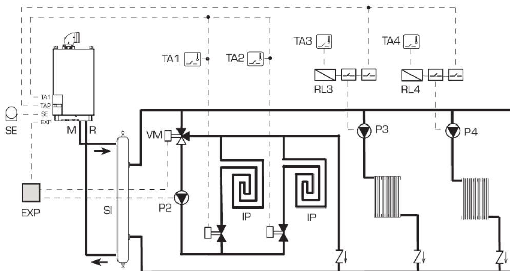
13. Systém s jedním směšovacím okruhem, 2 řízenými topnými větvemi a čidlem venkovní teploty (obj.č.8094101)
